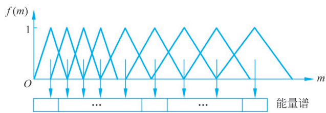
图 5-11 Mel 频率滤波器组
