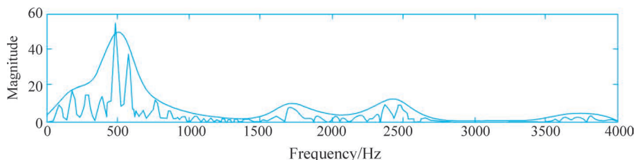
图 5-9 傅里叶变换后的频谱图
